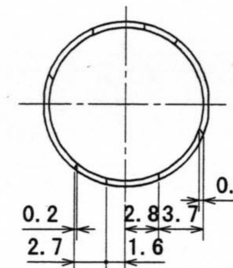
C-C 断面図
