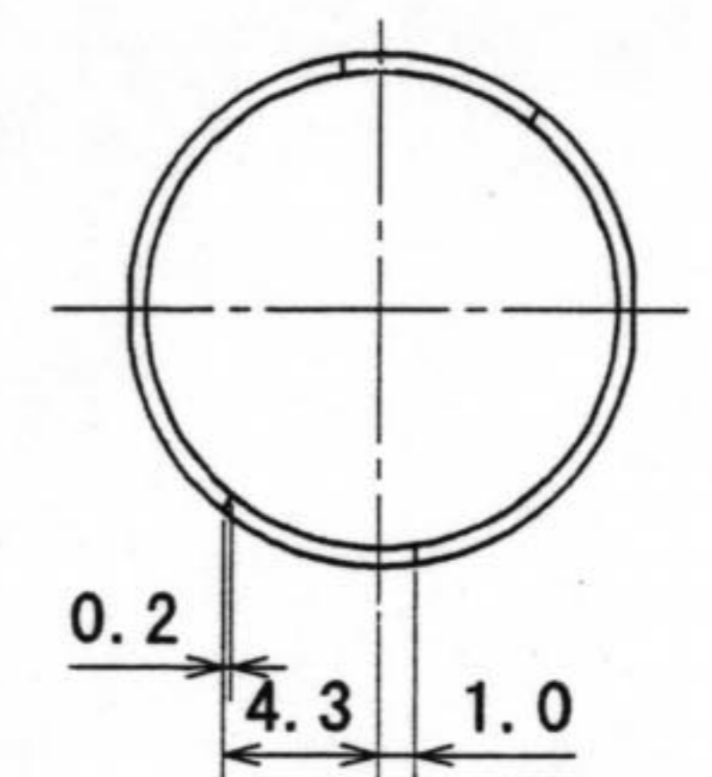
D-D 断面図
