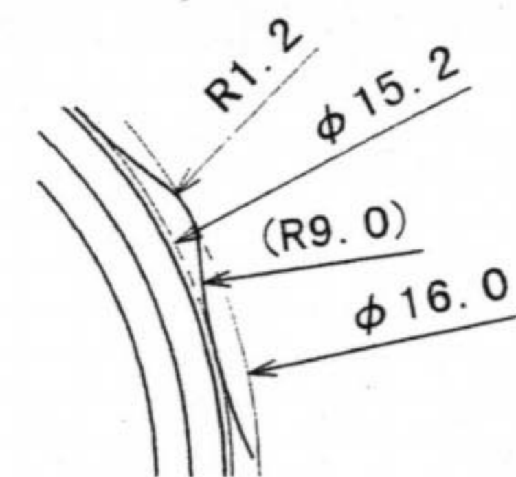
F部拡大図 5/1
