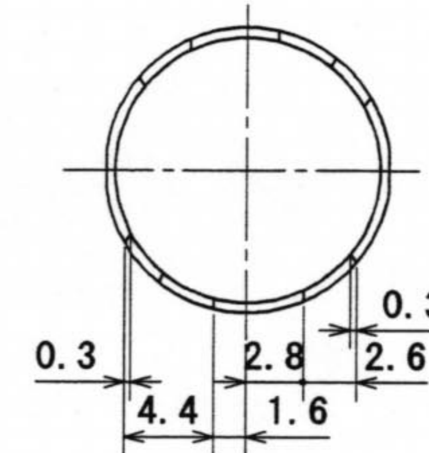
B-B 断面図
