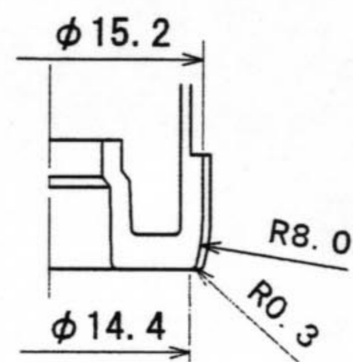
H-H 断面図
