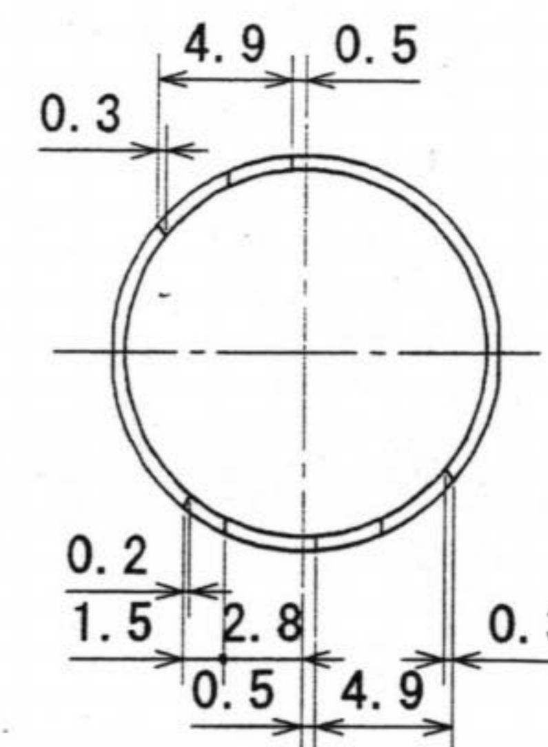
A-A 断面図
