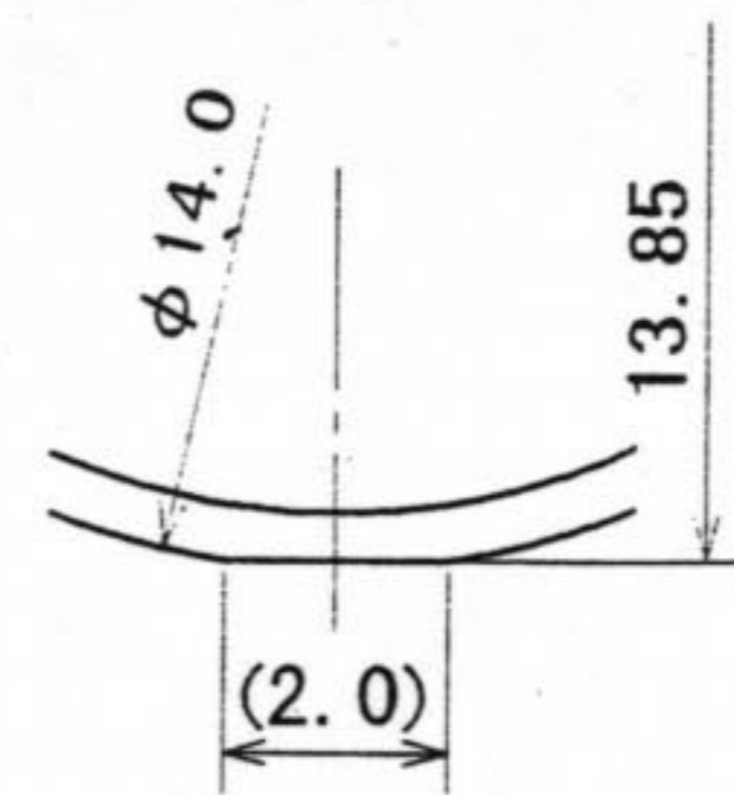
G-G 断面図拡大図 5/1
